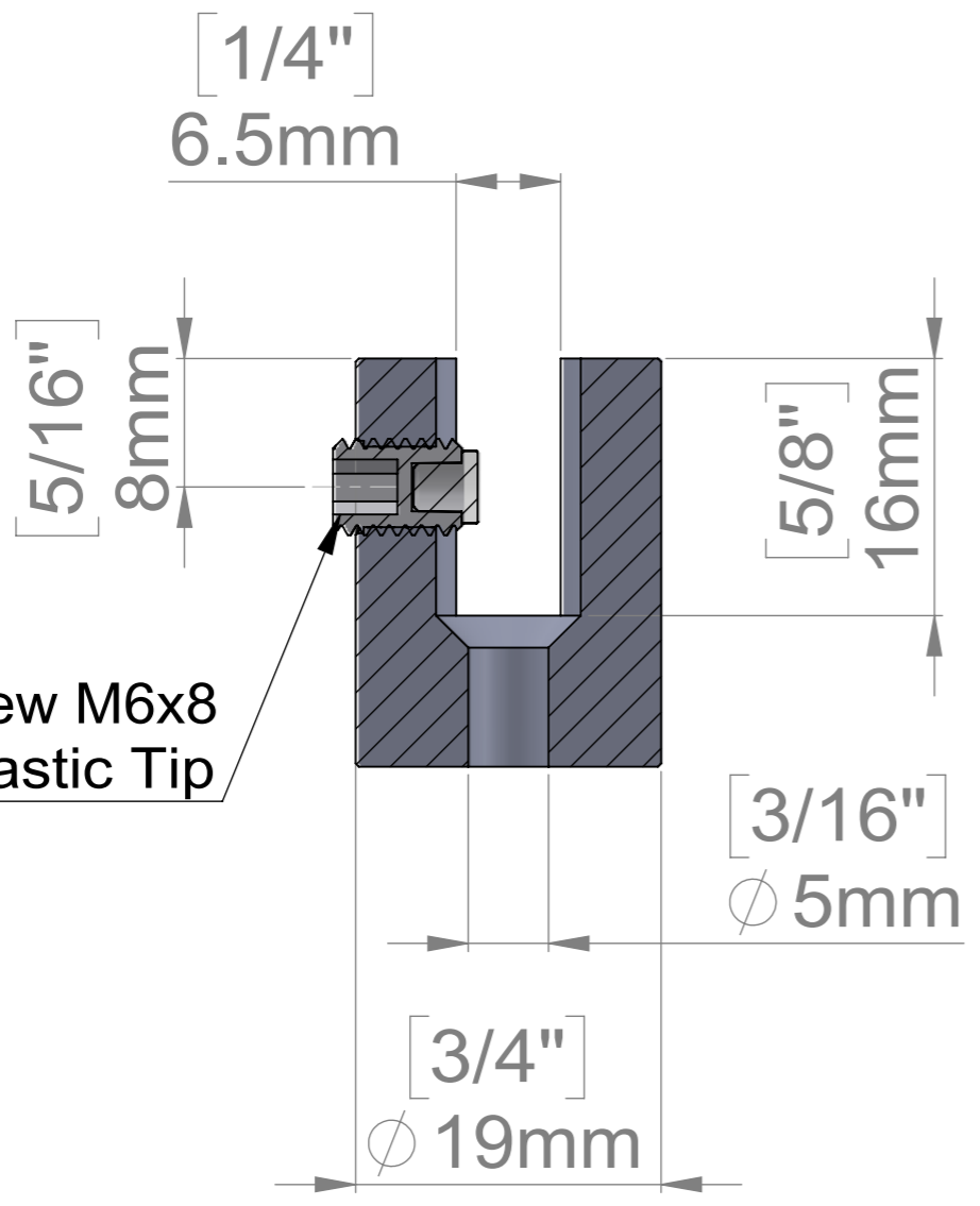
SECTION A-A
