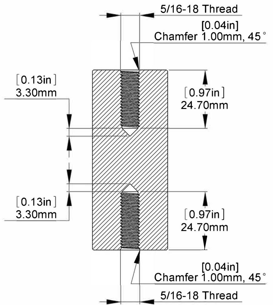
SECTION A-A
